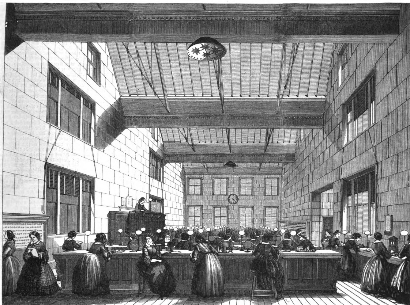
Der große Telegraphieraal im Gebäude der internationalen Telegraphengesellschaft in London.
