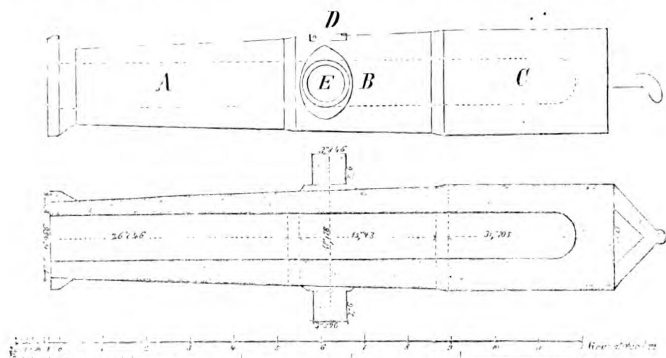
Noch einer sächsischen 12pfündigen Granatannon. Seitenansicht und Längendurchschnitt.
