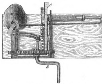
Amerikanischer Hebel- oder Kettenschleife von James Smith.
