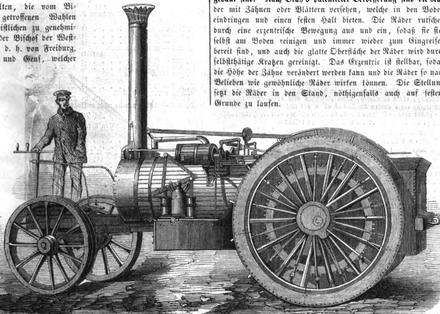
Bray's verbesserte Zugmaschine.
